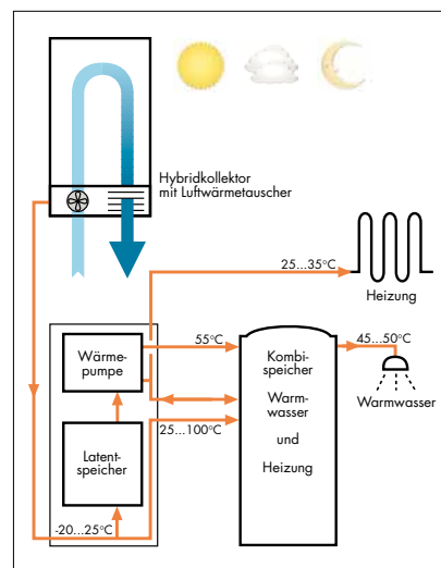
Das Solaera-Funktionsprinzip: Die Solarheizung liefert auch bei Schlechtwetter und nachts ausreichend Wärme.
